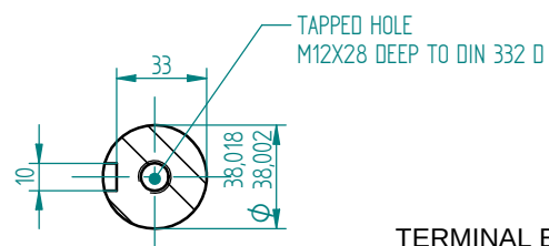
Przekrój A-A 1:2
